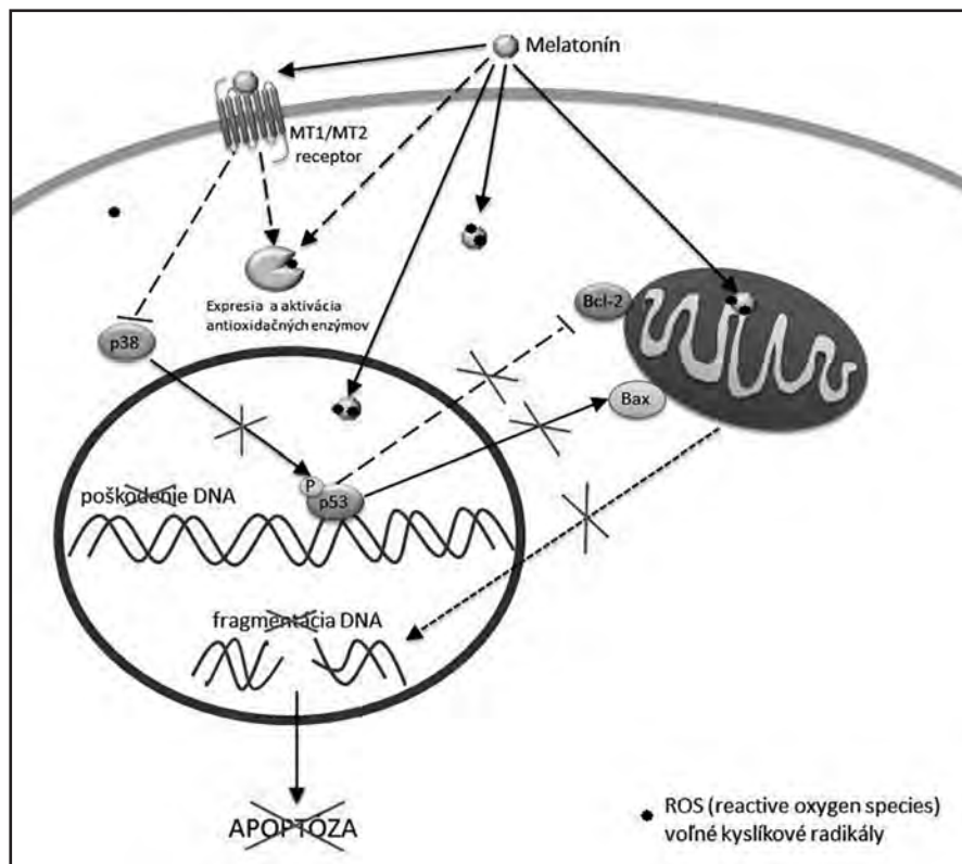
Obr. 3: Melatonin inhibuje vnútornú dráhu apoptózy v normálnych bunkách. Melatonin je schopný inhibovať vnútornú dráhu apoptózy v normálnych bunkách nepriamou inhibíciou p38 pomocou jeho receptor-závislej dráhy. Proteín p38 následne nie je schopný fosforylovať p53, a tým nedochádza k jeho transkripčnej aktivite a akumulácii v bunke. Melatonin taktiež zohráva úlohu ako vychytávač voľných radikálov v bunke a taktiež zvyšuje expresiu a aktivitu iných antioxidačných enzýmov.
